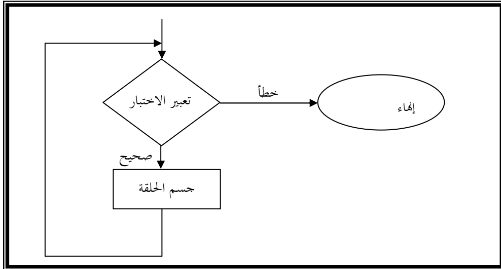
شكل (3-1) - طريقة عمل الحلقة while
